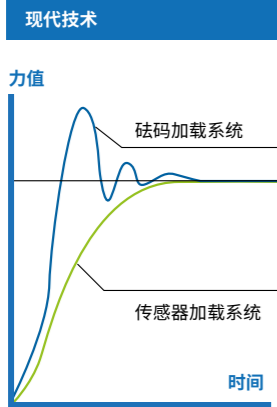
力传感器，闭环，力反馈系统
